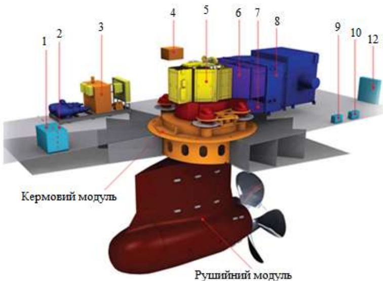
Рис. 3.1. Гребна електрична установка Azipod серії V:
