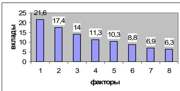
Рис. 7.2. Внески параметрів і ефектів взаємодій у показник \Delta\omega_D
