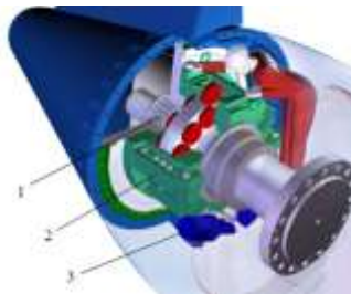
Рис. 3.12. Схема упорного підшипника установок "Azipod XO":
