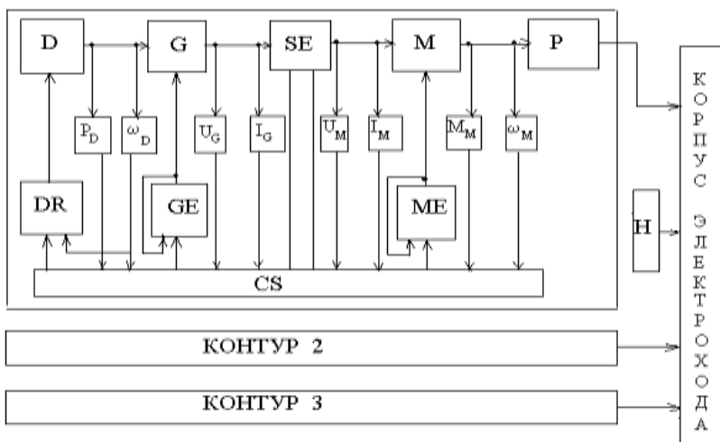
Рис. 6.1. Структурна схема пропульсивного комплексу електрохода
