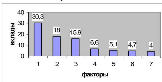
Рис. 6.6. Внески параметрів і ефектів взаємодій у показник (I_M)_{Tm}
