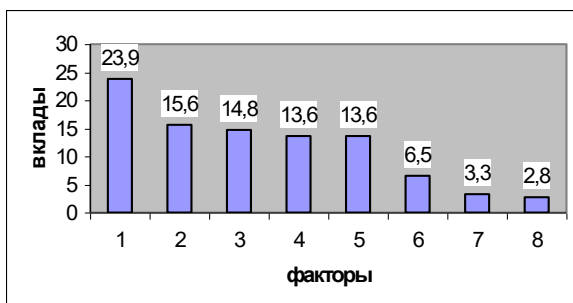
Рис. 7.3. Внески параметрів і ефектів взаємодій у показник (T_{CV})_{rev} .
