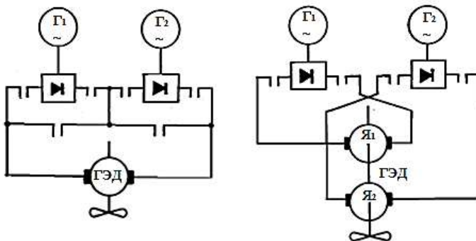
Рис. 2.5. Схеми головного струму для однажірних і двох-жірних ГЕД
