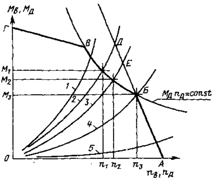
Рис. 1.4. Механічні характеристики: ГЕД – A-D ;
