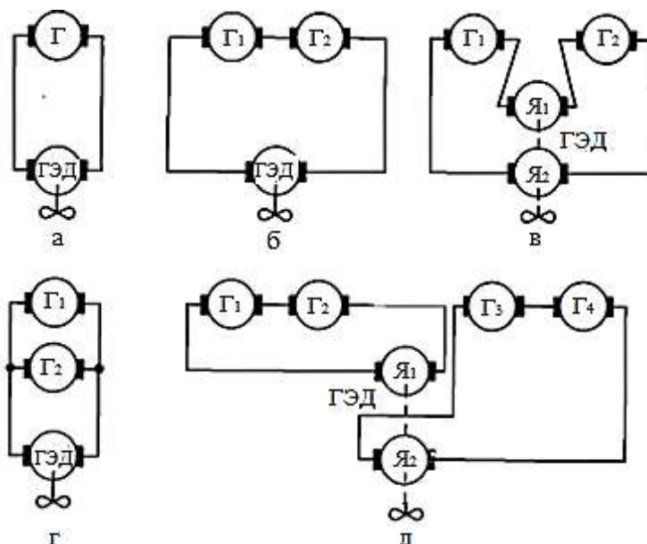
Рис. 2.4. Схеми головного струму одновальних ГЕУ
