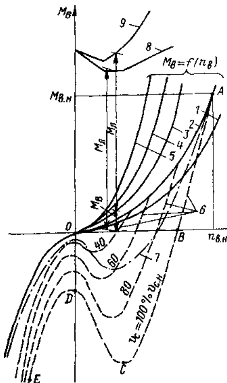
Рис. 1.2. Реверсивні характеристики гребного гвинта.
