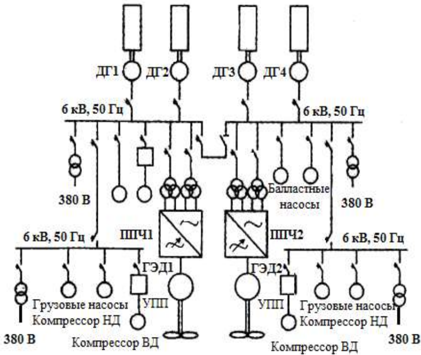
Рис. 2.12. Структурна схема ЄЕЕС танкера-газовоза:
