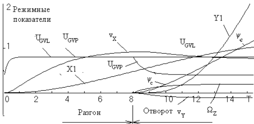
Рис. 6.8 а. Режимні показники силової установки електрохода з ГЕУ з частотно-керуваними ГЕД
