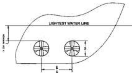
Рис. 5.6. Типове розташування ТПП, які працюють у тандемі (Lighest Waterline - ватерлінія під час плавання порожнім)
