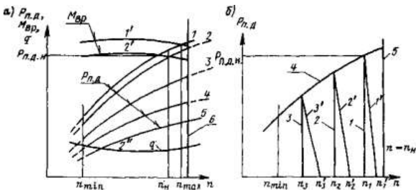
Рис. 1.3. Характеристики дизеля: а – швидкісні; б – регуляторні; в – навантажувальні
