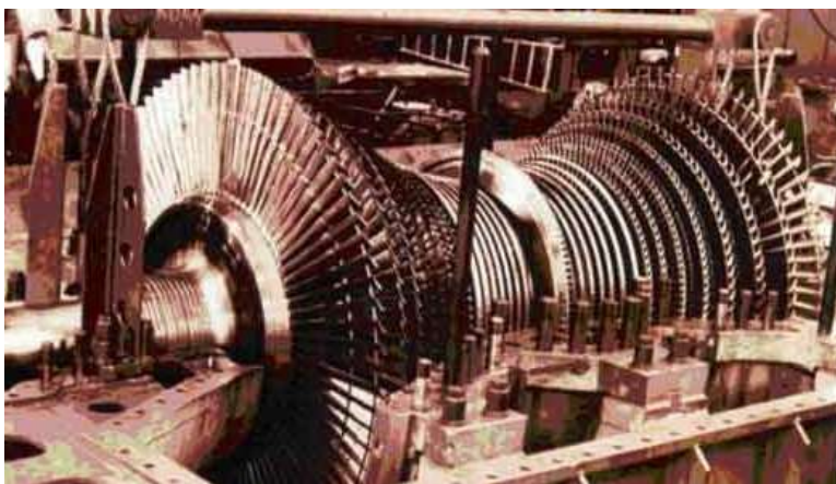
Рис. 2.8. Турбіна ГТА-642 атомного криголама «Арктика»
