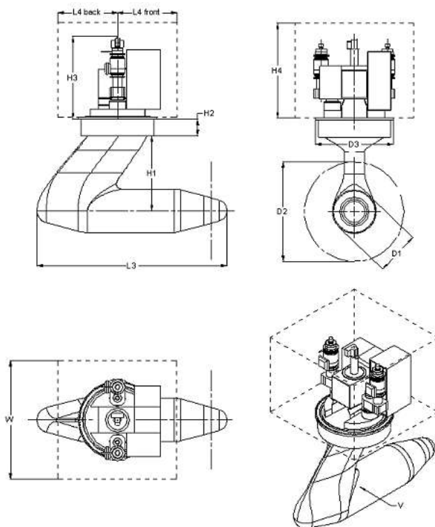
Рис. 3.16. Схема конструкції ГЕУ Azipod ® CO
