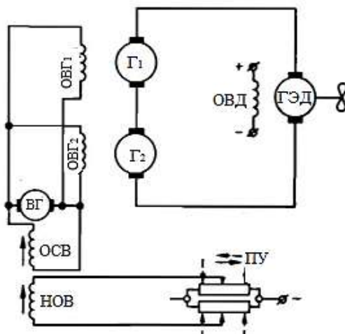
Рис. 2.3. Принципова схема ГЕУ:
