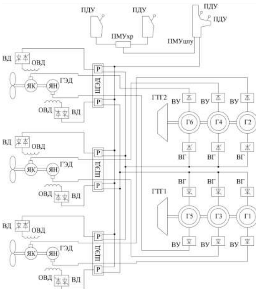
Рис. 2.7 Структурна схема ГЕУ криголаму «Арктика».
