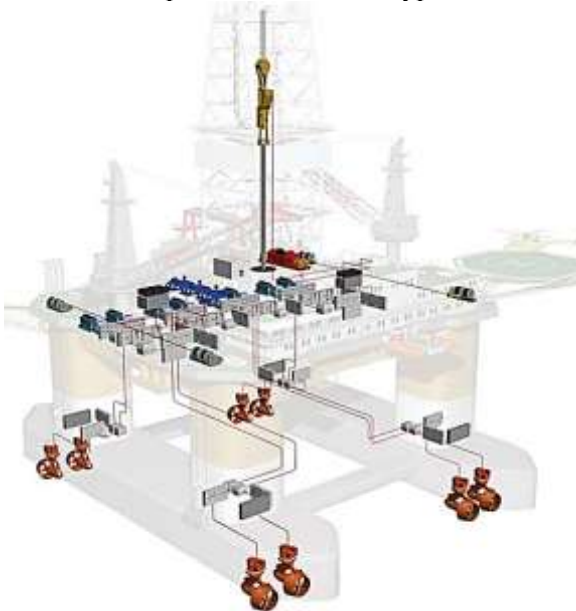
Рис. 3.18. Схема ГЕУ бурової платформи з установками Azipod® CZ
