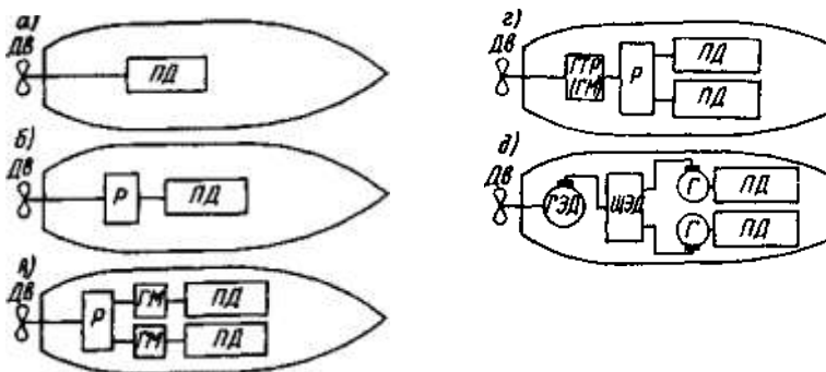
Рис. 1.1. Схеми передачі енергії від первинного двигуна до рушія.
