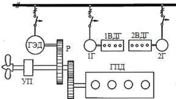
Рис. 2.1. Комбінована гребна установка траулера
