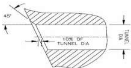
Рис. 5.8. Типовий вихідний отвір тунелю ТПП
